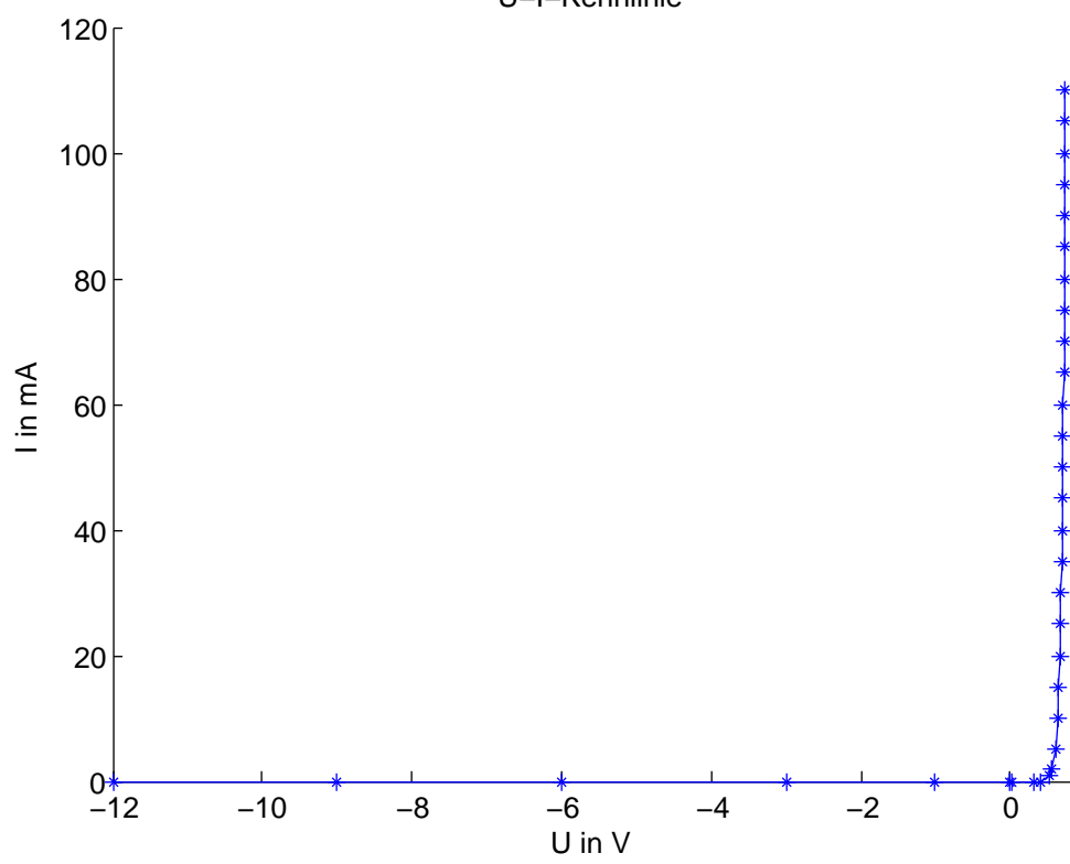
U-I-Kennlinie
