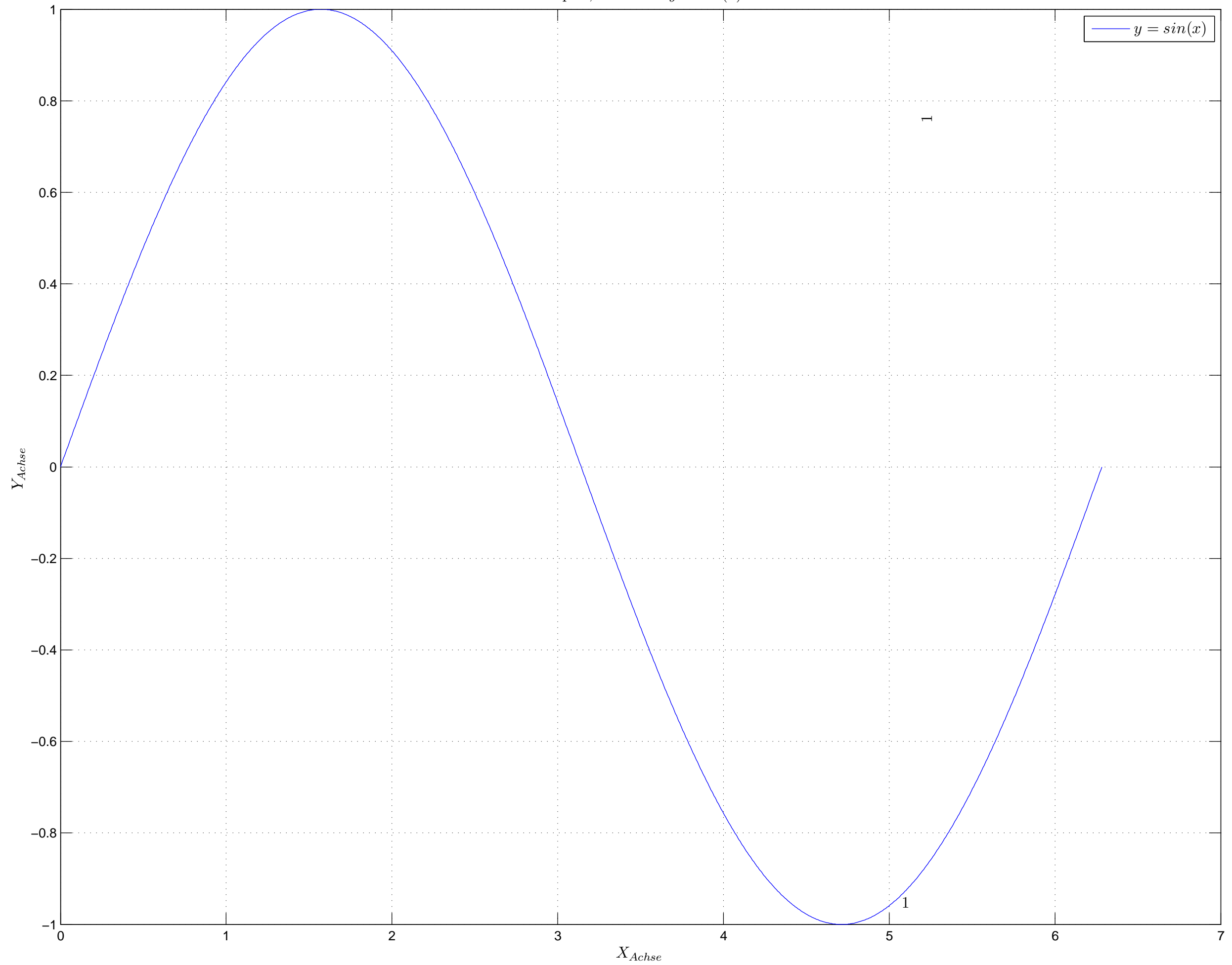
Testplot, Funktion: y = \sin(x)
