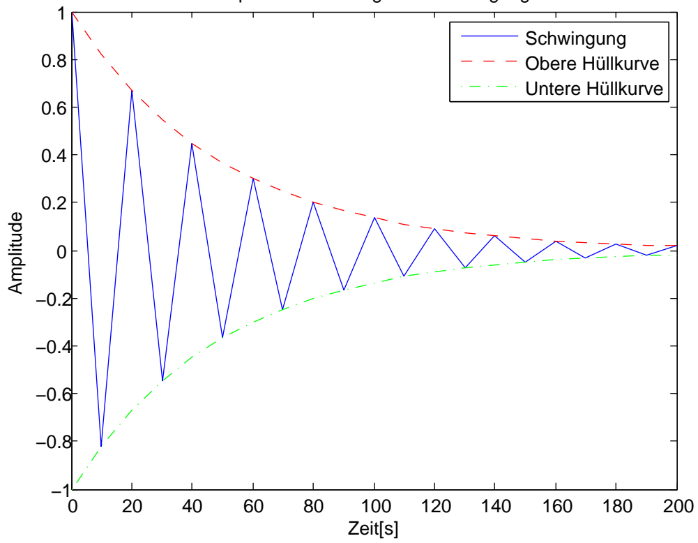
Exponentiell abklingende Schwingung
