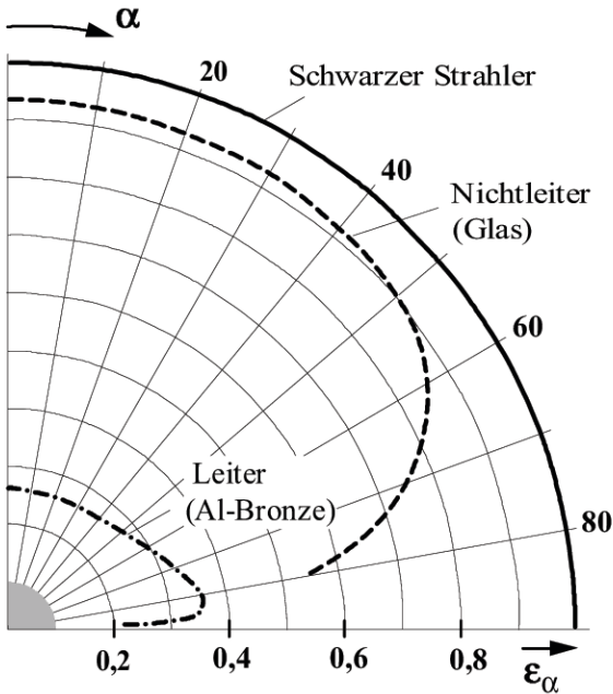
Abb. 8: Richtungsabhängigkeit des Emissionsgrades bei Leitern und Nichtleitern
